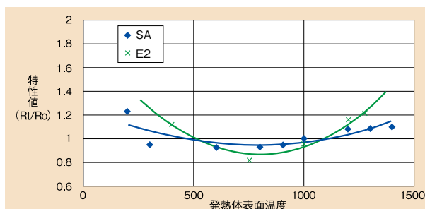
図3 SAの抵抗・温度特性
