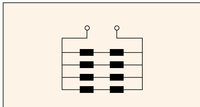
■図19 単相2本直列並列結線
