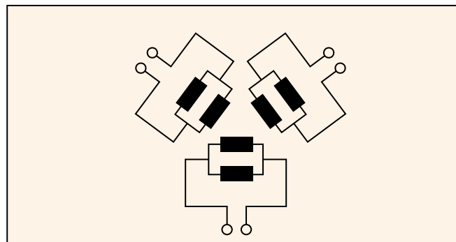
■図20 開放デルタ結線（単相3回路）
