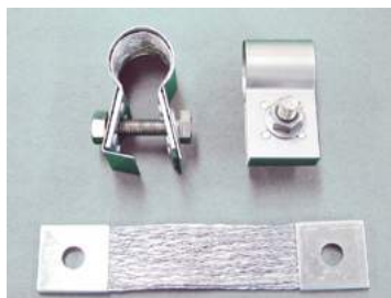
■耐熱締付型端子規格表
