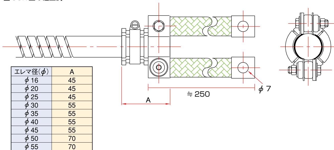
■ SGR 型の組立例
