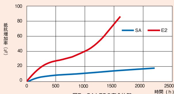
図5 SAとE2の寿命比較
