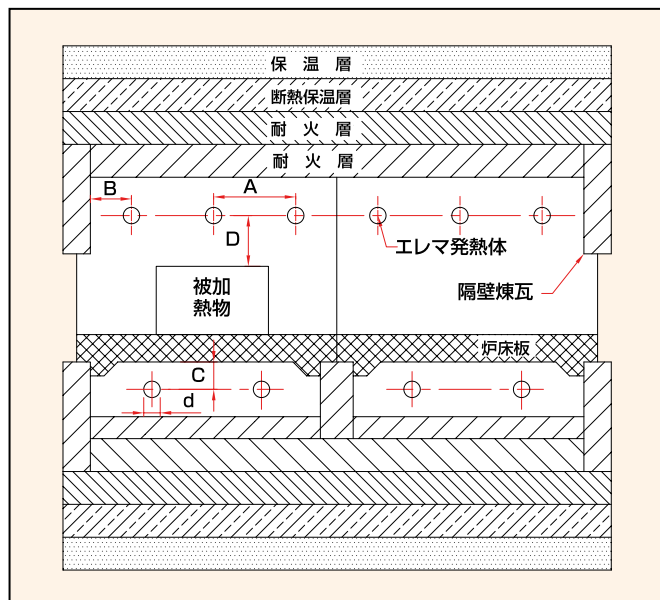
■図13 発熱体の取付間隔
