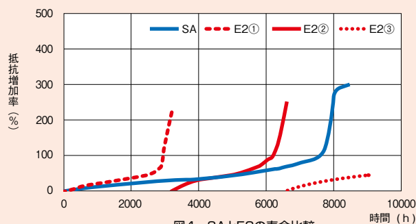
図4 SAとE2の寿命比較
